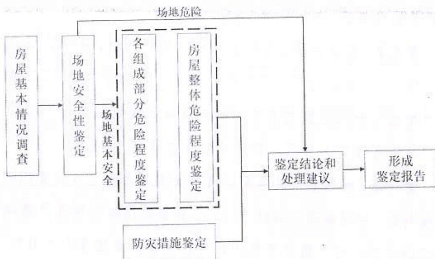
图 1 农村住房安全性鉴定程序
